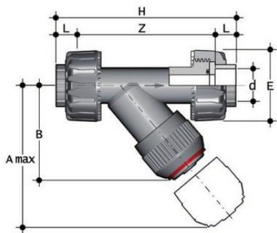
Грязевый фильтр RVUIV PBX с муфтовыми окончаниями, EPDM, FIP d16 (DN10)
