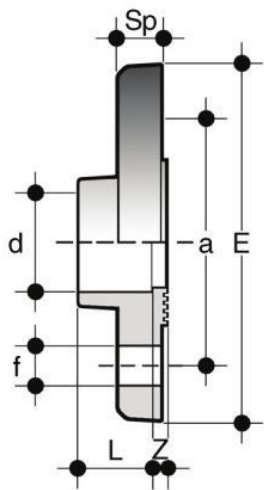
Жесткий фланец ПВХ FIP d75
