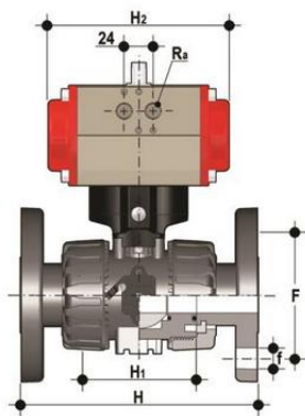
Шаровой кран VKD ХПВХ с пневмоприводом ДвД с фланцевыми окончаниями d50 (DN40)
