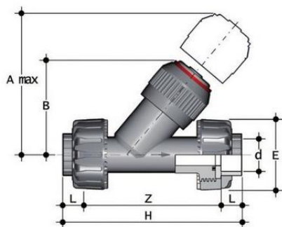
Угловой обратный клапан VRUIV ПБХ с разборными муфтовыми окончаниями, FKM, FIP d20 (DN15)
