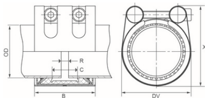
Соединительная муфта GRIP Ø54.0-168.3, EPDM, W5 d154
