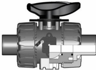
Шаровой кран ПВХ для регулирования потока VKR со втулочными окончаниями, FKM, FIP d20 (DN15)
