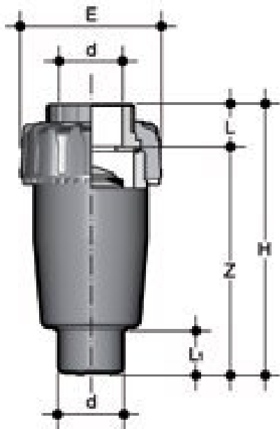
Воздухоотводный клапан VA ПВХ с муфтовыми окончаниями, EPDM, FIP d32 (DN25)
