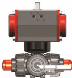
3-х ходовой шаровой кран ТКД с пневмоприводом ДвД с муфтовыми окончаниями, L-шар (уплотнение EPDM) PP-H d32 (DN25)
