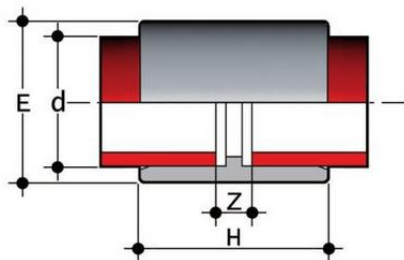
Муфта соединительная PP-H FIP d63 PN10
