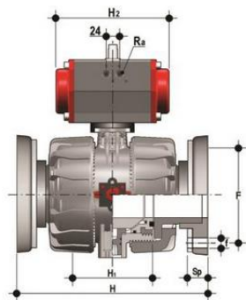
Шаровой кран VKD с пневмоприводом H3 с фланцевыми окончаниями, DN65-100 (уплотнение FKM) PP-H d75 (DN65)
