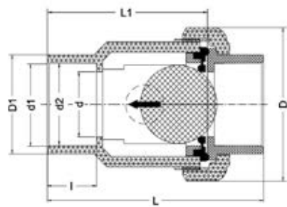
Шаровой обратный клапан с одним разборным окончанием ISR ПВХ; с муфтовыми окончаниям, EPDM, IPS d75 (DN65)
