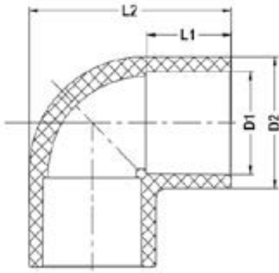
Отвод 90° ХПВХ IPS (Model A) d50 PN16
