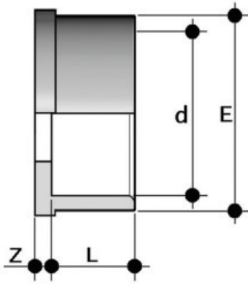
Муфтовое окончание для ВIV ПВХ FIP d16
