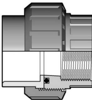
Муфта разборная с ВР ПВХ FIP 110x4
