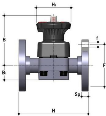
Мембранный клапан ДК ПВДФ с фланцевыми окончаниями d50 (DN40)
