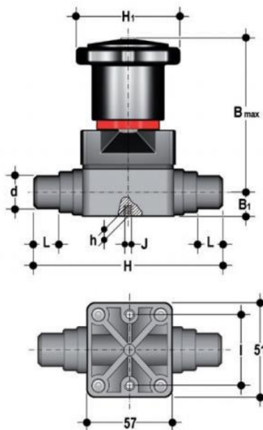
Компактный мембранный клапан CMDC ХПВХ с втулочными окончаниями d20 (DN15)
