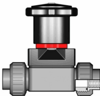
Компактный мембранный клапан ПВХ с пневмоприводом, CM, FKM, FIP R1/2" (DN15)
