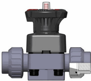
Мембранный клапан DKUFV ПВХ с резьбовыми окончаниями, EPDM, FIP R1" (DN25)
