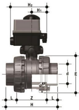
Шаровой кран VXE ПВХ с пневмоприводом ДвД с муфтовыми окончаниями, FKM, FIP d75 (DN65)
