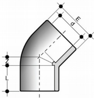
Отвод клеевой 45° ПВХ FIP d75
