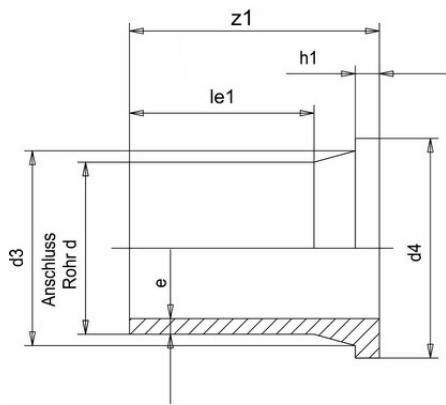
Бурт PP-H Simona d250 SDR11 PN6
