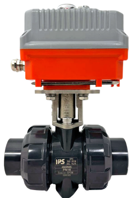
Шаровой кран IVKD ПВХ с эл.приводом (площадка IPQ) 220V, муфтовые окончания, EPDM, IPS d20 (DN15)
