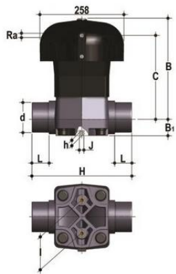
Мембранный клапан VM ПВХ с пневмоприводом НЗ, втулочные окончания, EPDM, FIP d90 (DN80)
