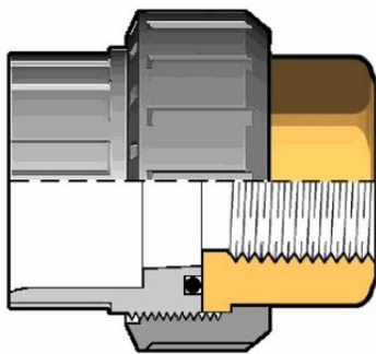
Муфта разборная с ВР ПВХ (латунь) FIP 63x2
