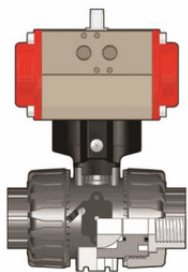
Шаровой кран VKD с пневмоприводом H3 с резьбовыми окончаниями (уплотнение EPDM) PP-H R2" (DN50)
