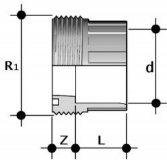
Муфтовая вставка для VIV PBX FIP d25
