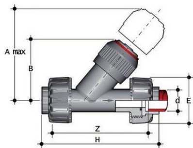
Угловой обратный клапан VR с муфтовыми окончаниями (уплотнение EPDM) PP-H d63 (DN50)
