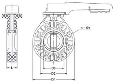
Дисковый затвор IFK ПВДФ с рукояткой d225 (DN200)
