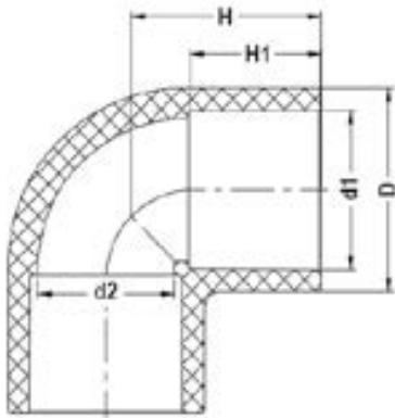
Отвод ПВДФ 90° (IPS) d90 PN 16
