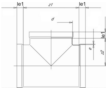
Тройник равнопроходной PPs d63
