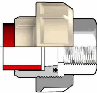
Муфта разборная переходная PP-H / нерж.сталь, ВР, (FKM) FIP 20x1/2 PN10
