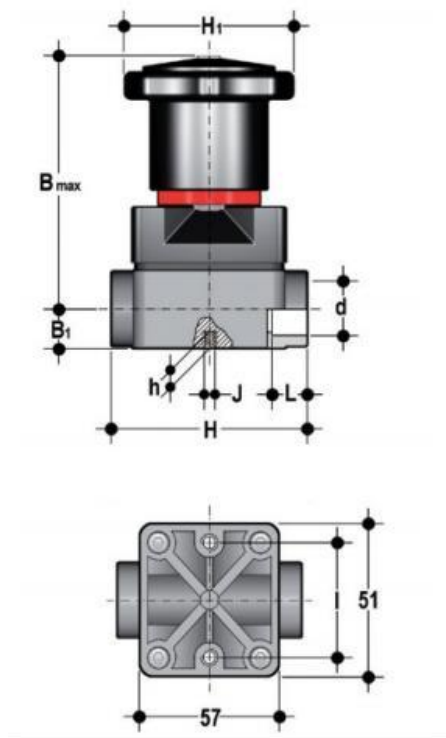
Компактный мембранный клапан CMIV ПВХ с муфтовыми окончаниями, EPDM, FIP d20 (DN15)
