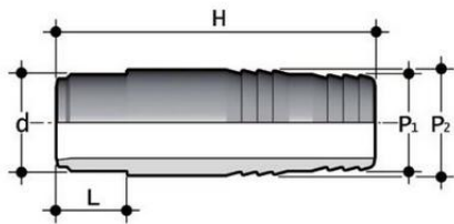
Шланговый адаптер PP-H FIP d25 PN10
