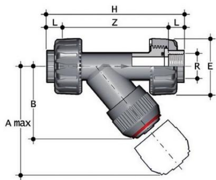
Грязевый фильтр RVUFT PBX с резьбовыми окончаниями, EPDM, FIP R1½" (DN40)
