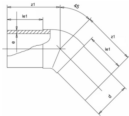
Отвод ПВДФ 45° (Simona) d50 SDR21 PN16
