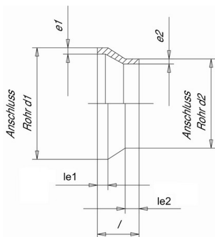
Муфта редукционная PP-H Simona (PN10) 75x40 SDR11 PN10
