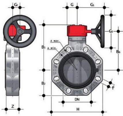
Дисковый затвор ПВХ FKOVRM с редуктором, FKM, FIP d225 (DN200)
