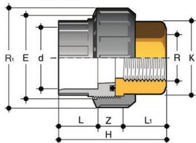
Муфта разборная с ВР ПВХ (латунь) FIP 50x1½"
