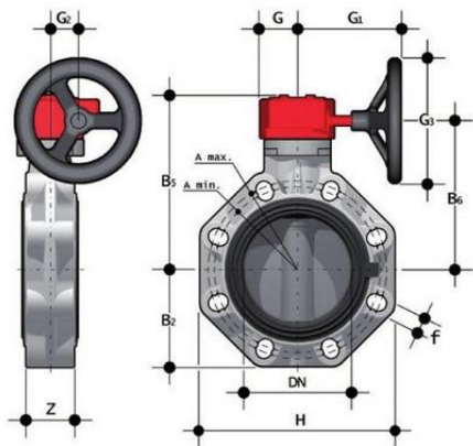
Дисковый затвор ПВХ FKOVRM с редуктором, EPDM, FIP d75 (DN65)
