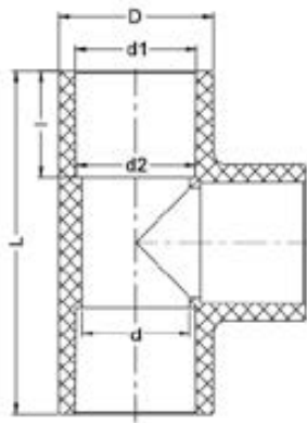
Тройник 90° ХПВХ IPS (Model A) d32 PN16
