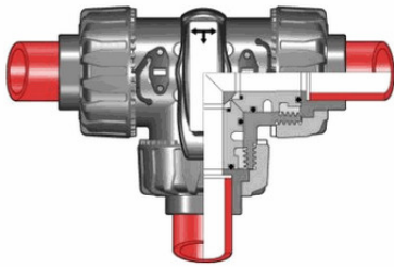
3-х ходовой шаровой кран ТКД с муфтовыми окончаниями L-шар (уплотнение EPDM) PP-H d32 (DN25)
