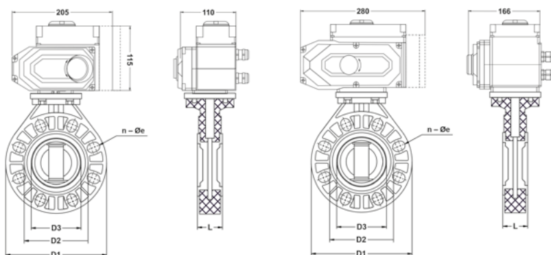
DN 50-125
